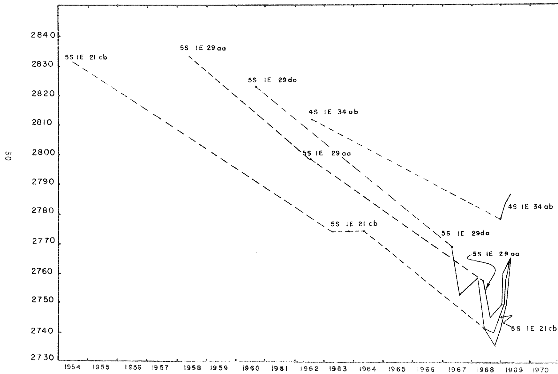
FIGURE 15. Hydrographs of wells 4S 1E 34ab1, 5S 1E 21cb, 5S 1E 29aa and 5S 1E 29da in the Oreana Subarea
